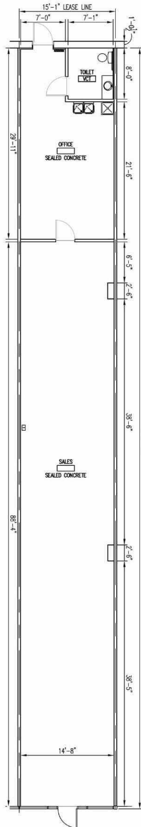
FLOOR PLAN SCALE: 1/8" = 1'-0"
